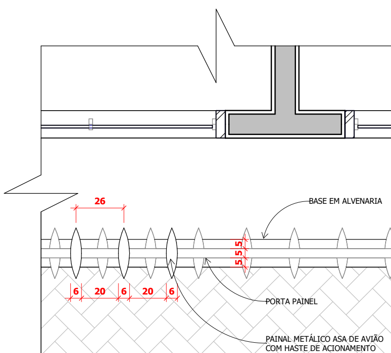
5 Detalhe Brise - Planta ESCALA 1:20
