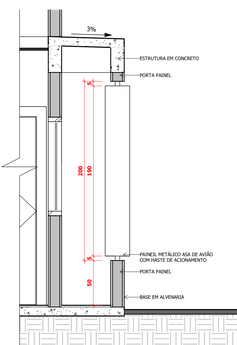
7 Detalhe Brise - Corte ESCALA 1:25
