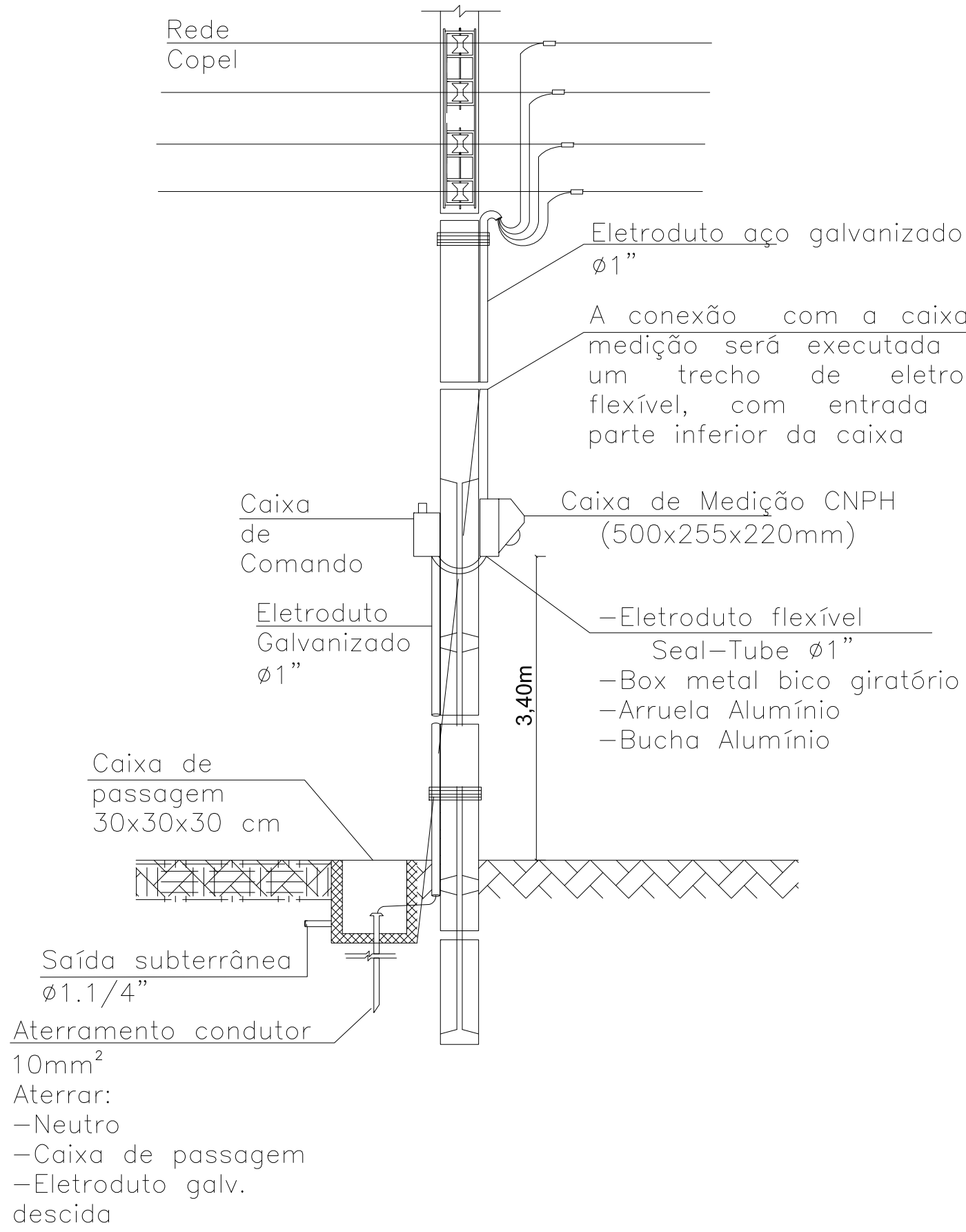
MEDIÇÃO E COMANDO EM POSTE COPEL
