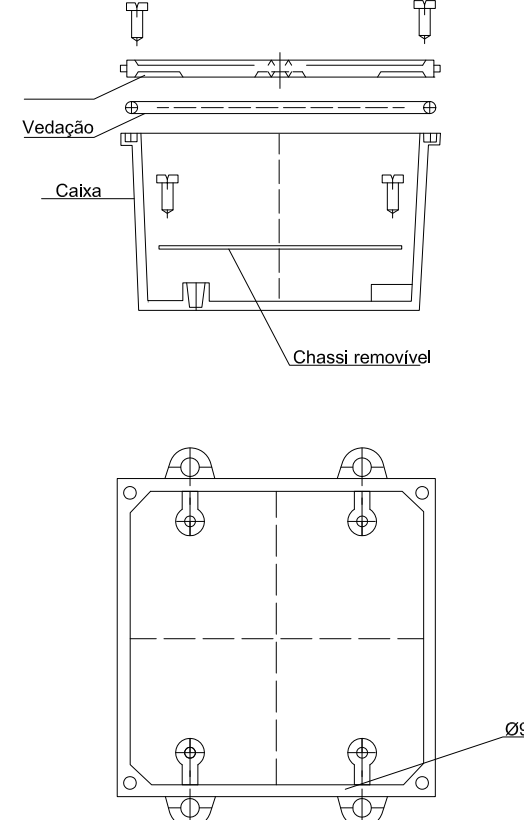
DETALHES CAIXA DE PASSAGEM COM TAMPA ANTIDERRAPANTE - UMA EM CADA POSTE
