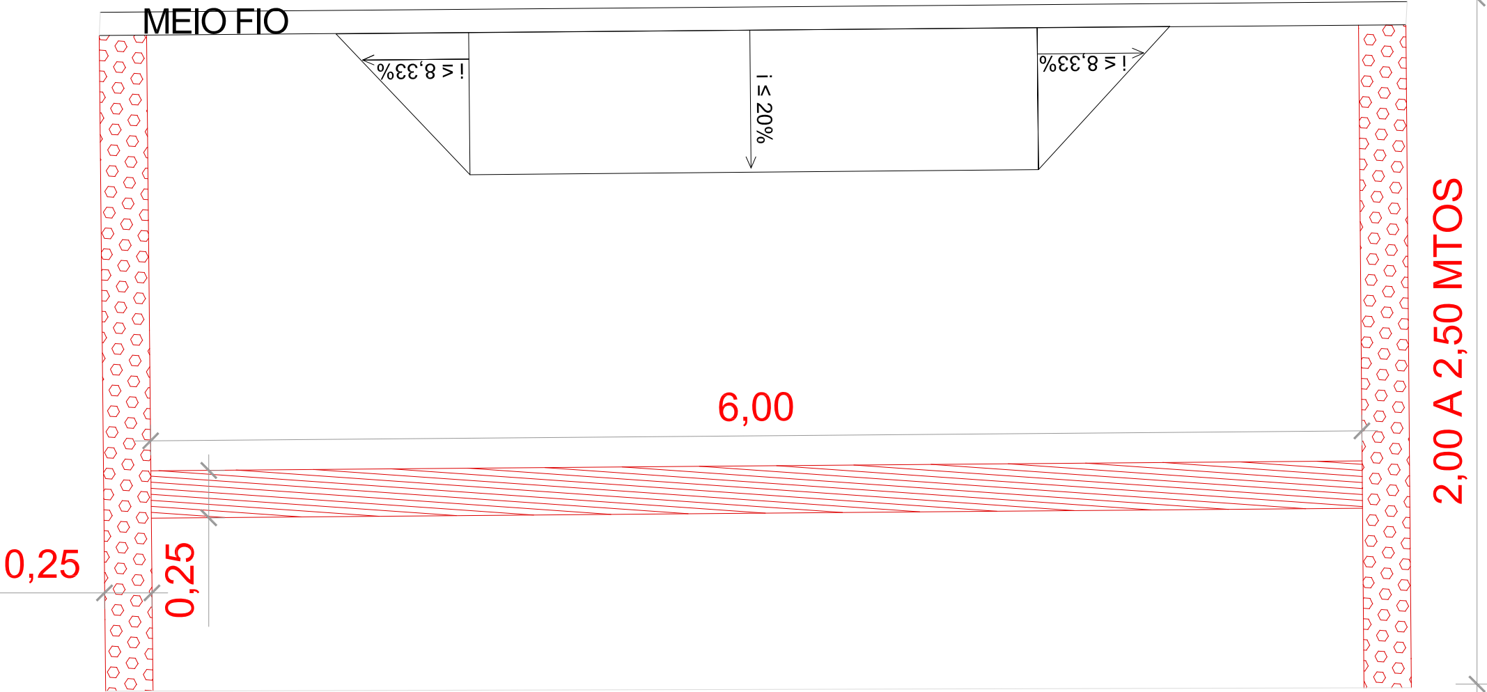
DETALHE ACESSO DE VEÍCULOS S/ Escala
