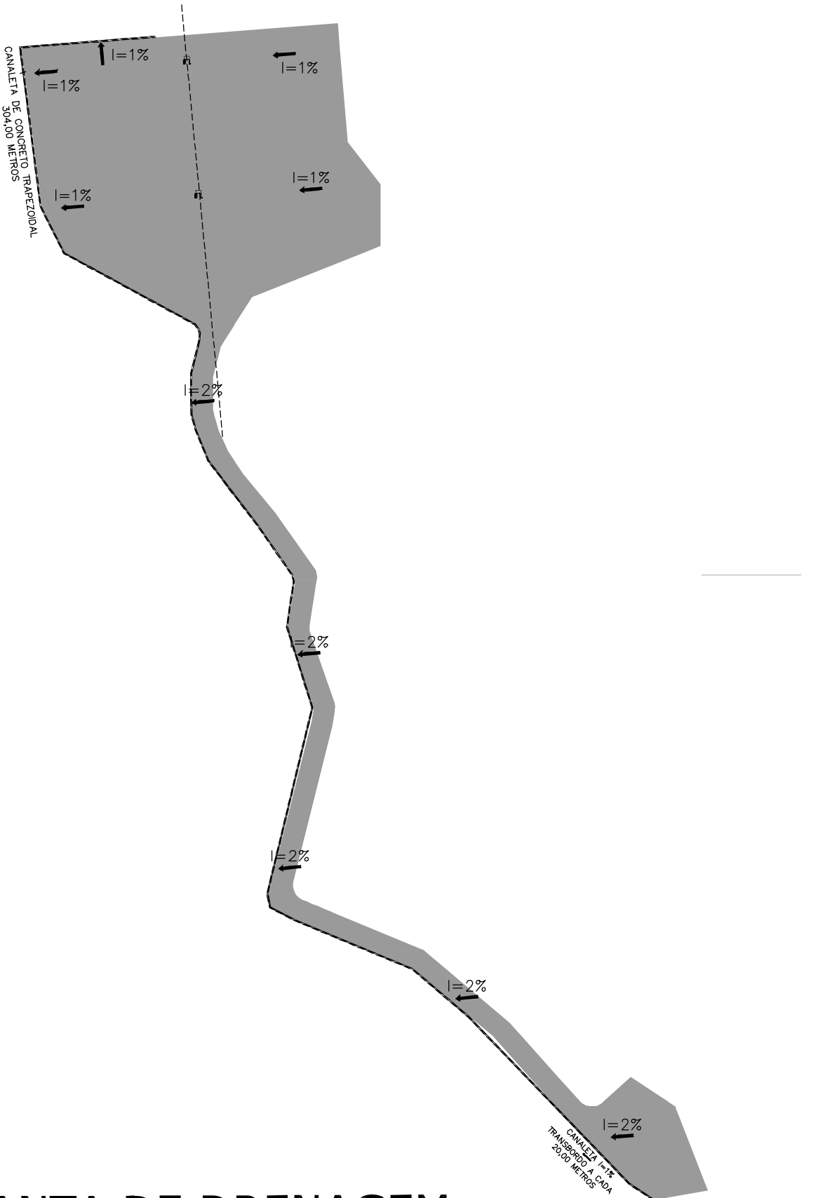
PLANTA DE DRENAGEM ESCALA 1/1000
