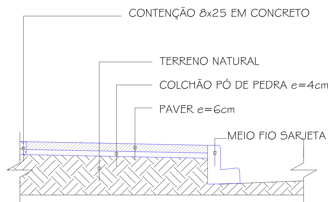
CORTE GENÉRICO CALÇADA S/ Escala
