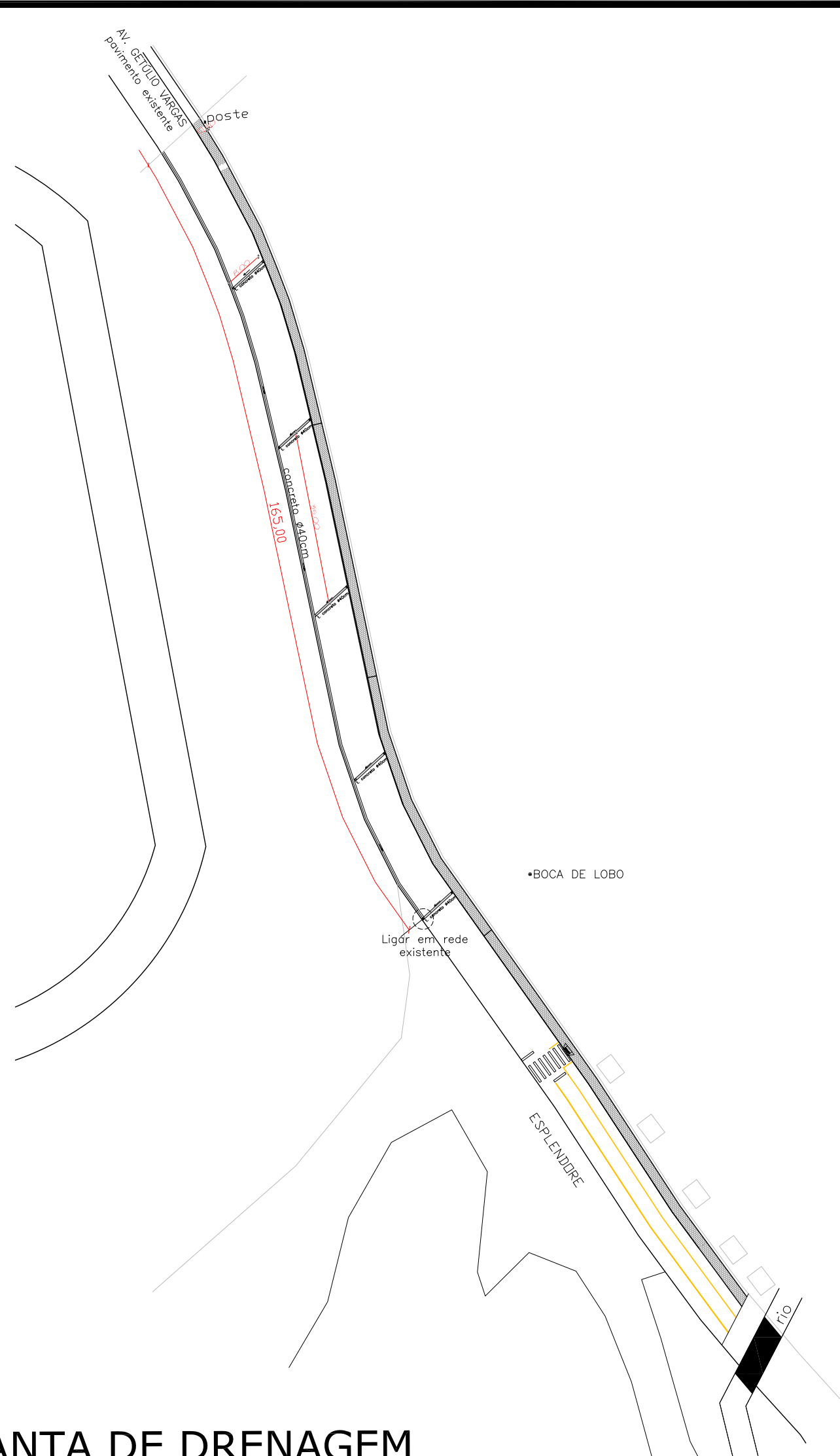
PLANTA DE DRENAGEM ESCALA 1/1000
