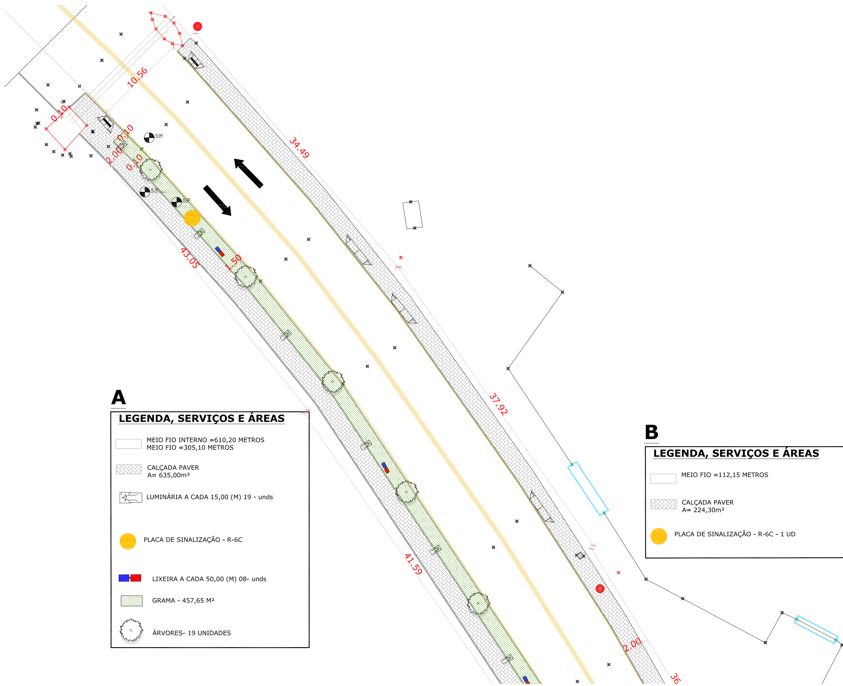
PLANTA DE SINALIZAÇÃO E URBANIZAÇÃO- DETALHE ESC 1/250
