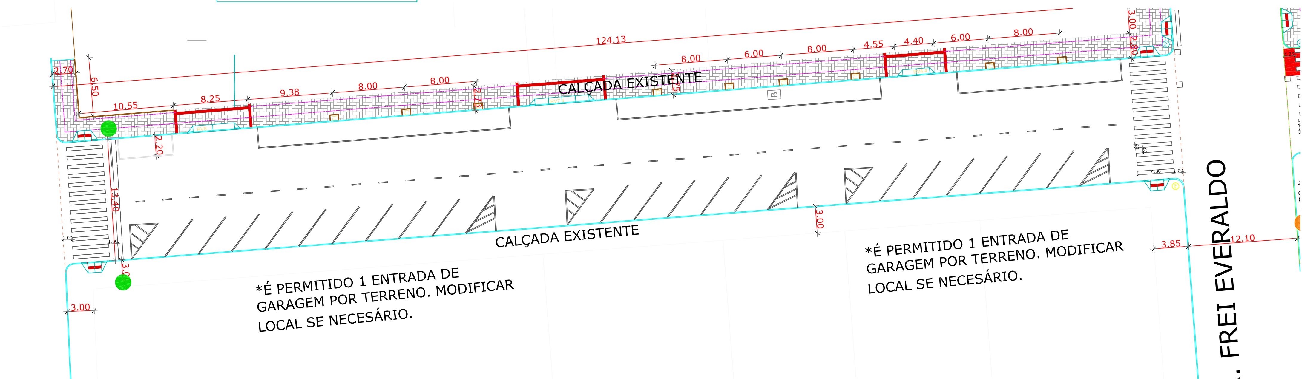
SINALIZAÇÃO RUA PRESIDENTE DUTRA ESC 1/250
