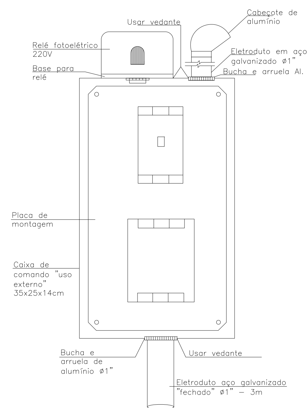
DETALHE CAIXA DE COMANDO
