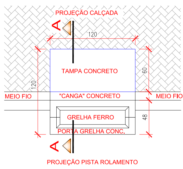
EM VISTA SUPERIOR
