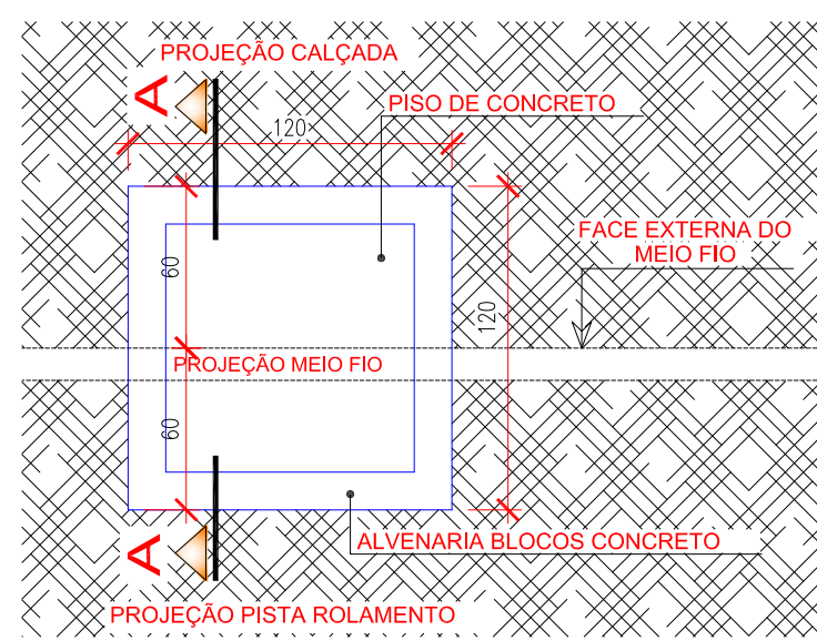
EM PLANTA
