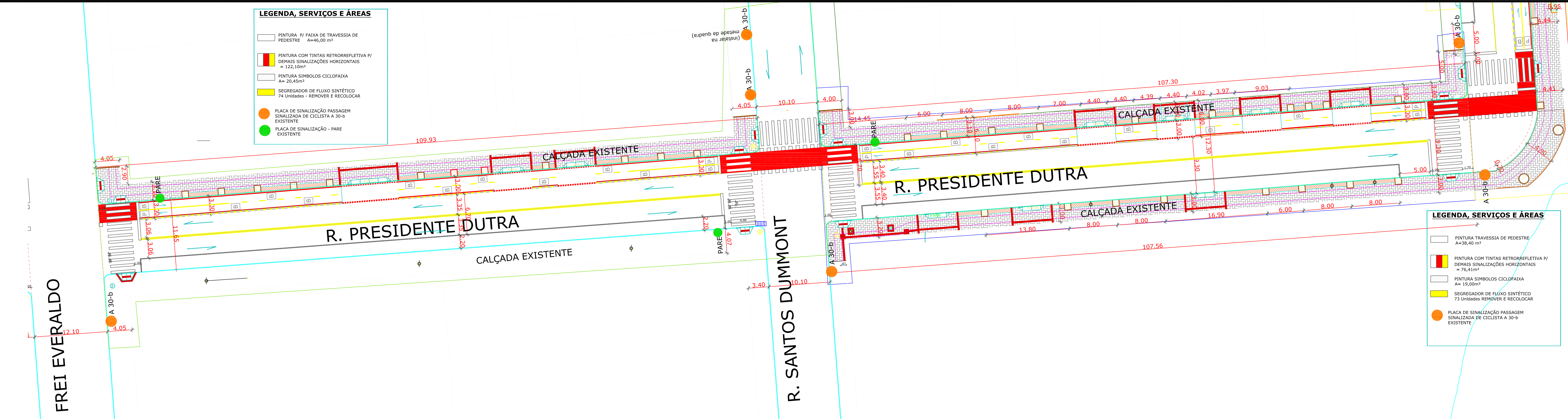
SINALIZAÇÃO RUA PRESIDENTE DUTRA ESC 1/250
