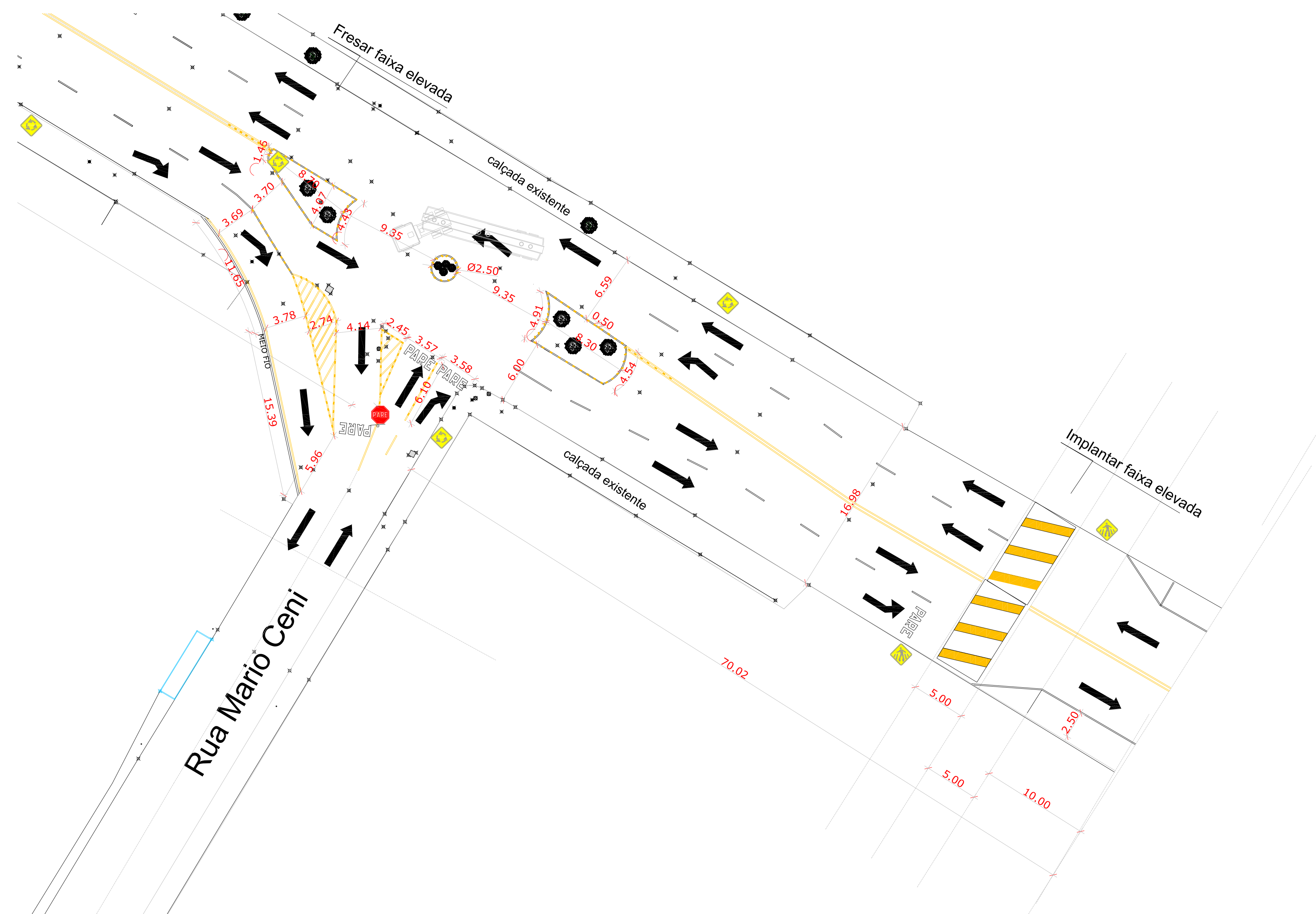
PLANTA DE SINALIZAÇÃO E URBANIZAÇÃO- DETALHE ESC 1/250
