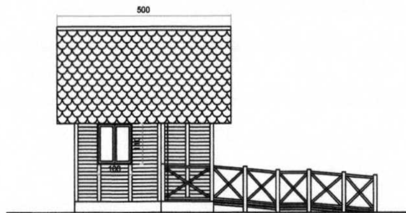
Fachada Lateral
