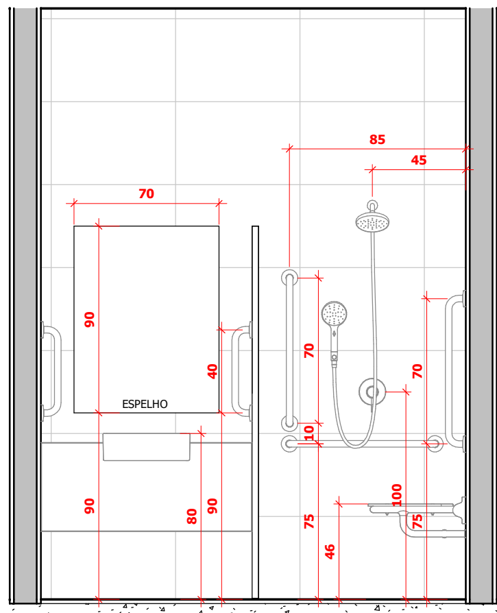
03 Vista 01 ESCALA 1:25
