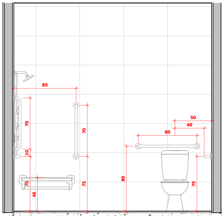
04 Vista 02 ESCALA 1:25
