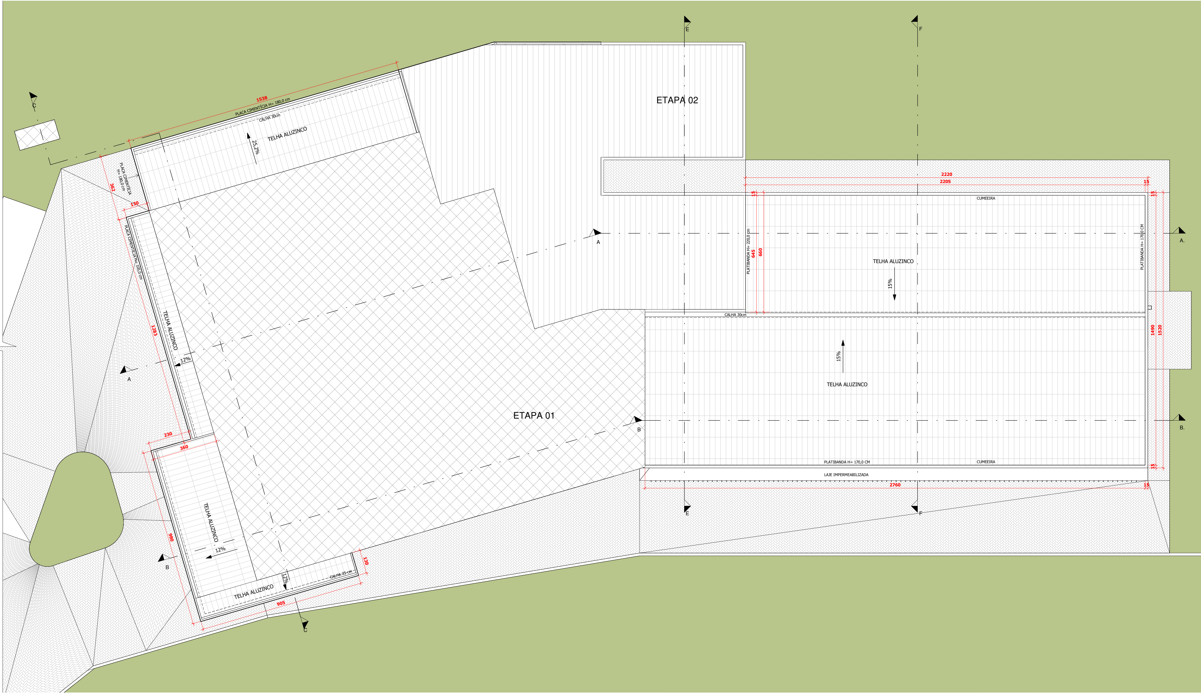
01 Cobertura ESCALA 1:100
